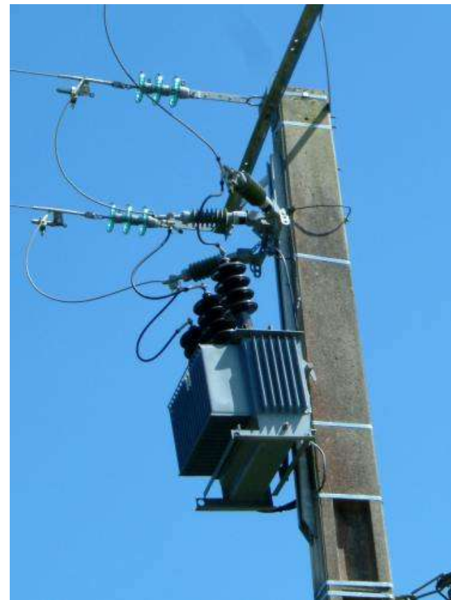
Eclateurs à cornes d'accrochage d'arc
