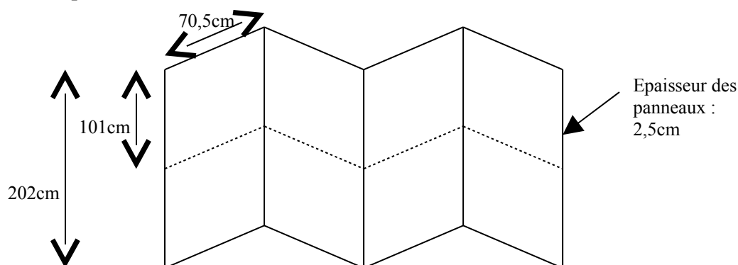
Schéma et dimensions du paravent
